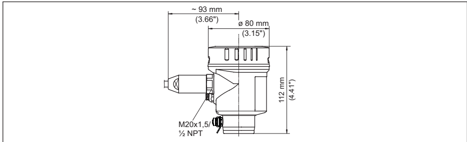
Fig. 31: Variantes de carcasa en grado de protección IP 66/IP 68 (1 bar), (con módulo de visualización y configuración integrado aumenta la altura de la carcasa en 9 mm/0.35 in)
