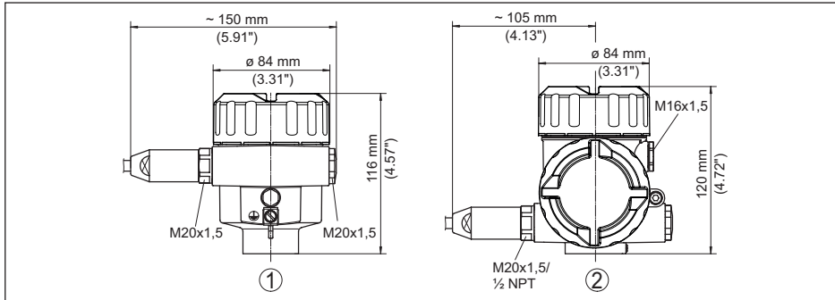
Fig. 29: Variantes de carcasa en grado de protección IP 66/IP 68 (1 bar), (con módulo de visualización y configuración integrado aumenta la altura de la carcasa en 9 mm/0.35 in)
