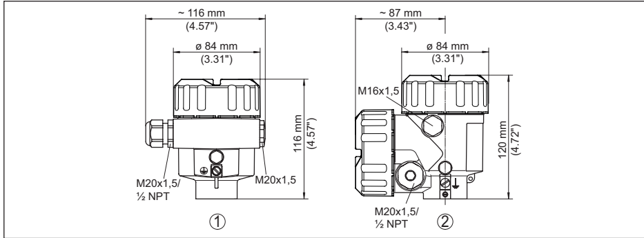
Fig. 28: Variantes de carcasa en grado de protección IP 66/IP 68; (0,2 bar), (con módulo de visualización y configuración integrado aumenta la altura de la carcasa en 9 mm/0.35 in)
