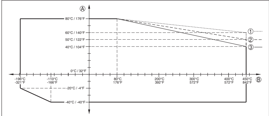
Fig. 25: Temperatura ambiente - Temperatura de proceso, versión estándar
