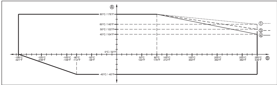
Fig. 24: Temperatura ambiente - Temperatura de proceso, versión estándar
