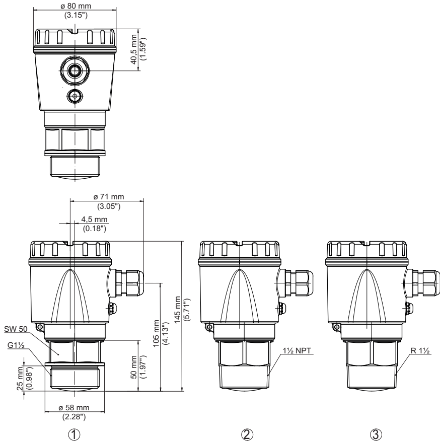
Fig. 7: Encombrement NivoRadar 7100
