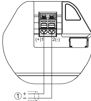
Fig. 19: Compartiment de raccordement NivoRadar 7100
