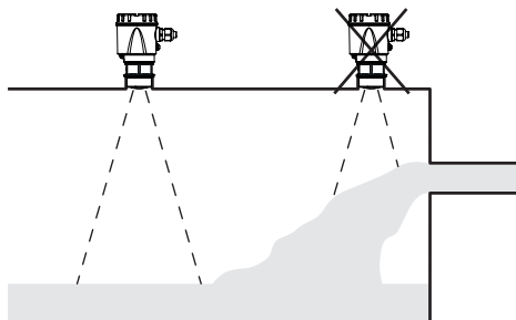
Fig. 12: Montage du capteur radar en présence d'un flux de produit
