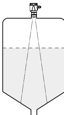
Fig. 10: Montage du capteur radar dans des cuves à fond conique
