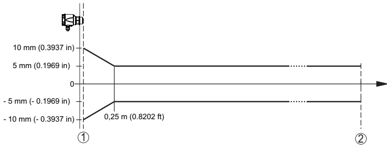
Fig. 6: Écart de mesure sous conditions de référence 1)
