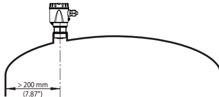
Fig. 9: Montage du capteur radar dans une cuve à toit bombé
