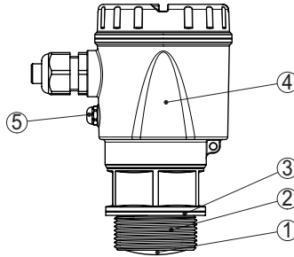
Fig. 1: Composants du NivoRadar 7100
