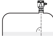
Fig. 16: Orientation du capteur dans les liquides
