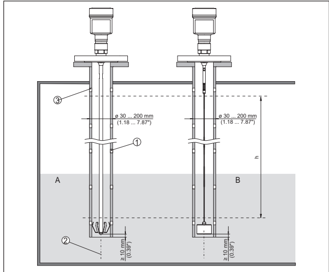
插图. 10: 安装在一根立管中
