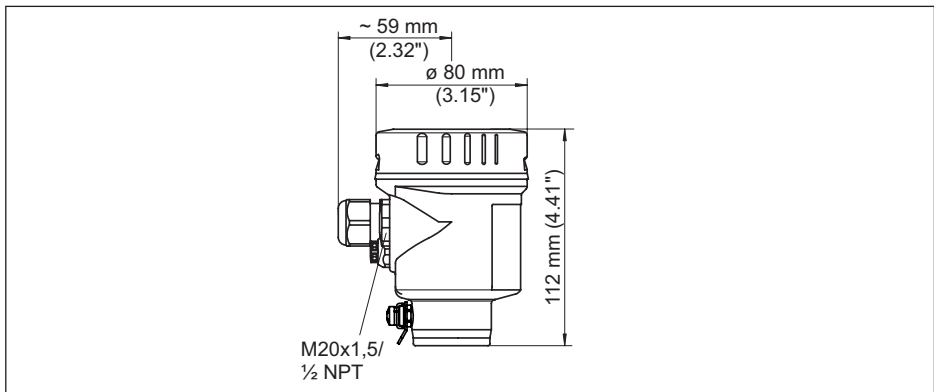
插图. 36: 采用保护等级达 IP 66/IP 68 (0.2 bar) 的壳体型式, (内装显示和调整模块后, 壳体高度增加了 9 mm/0.35 in)
