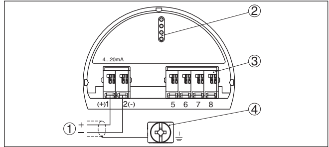
插图. 14: 单腔式壳体的电子部件和接线腔
