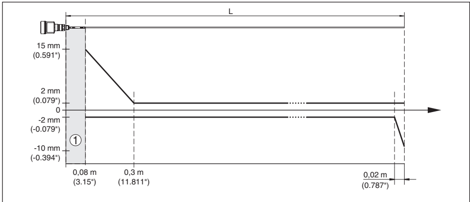
插图. 26: 棒型 NivoGuide 8100 在介质“水”中的测量偏差
