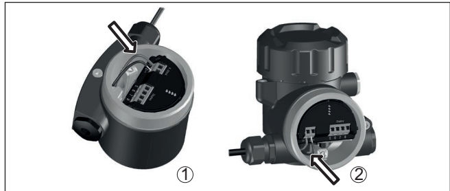
插图. 13: 接线步骤5和6
