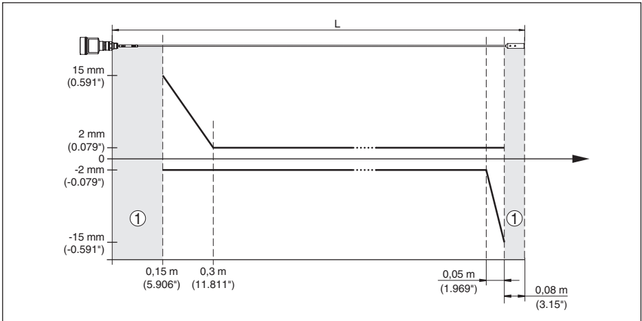
插图 29: 绳型 (∅ 2 mm/0.079 in) NivoGuide 8100 在介质“油”中的测量偏差
