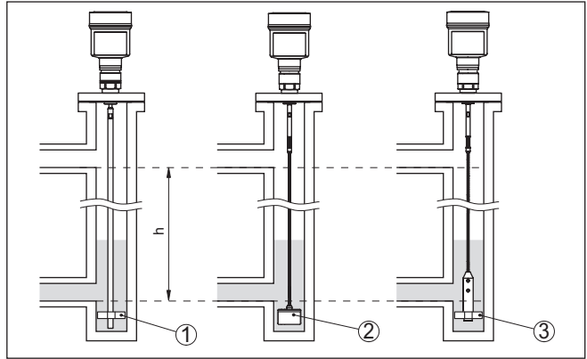
插图. 9: 安装在一根旁路管中 - 星形对中件或定心锤的位置
