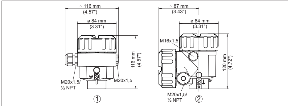
插图. 35: 采用保护等级达 IP 66/IP 68 (0.2 bar) 的壳体型式, (内装显示和调整模块后, 壳体高度增加了 9 mm/0.35 in)
