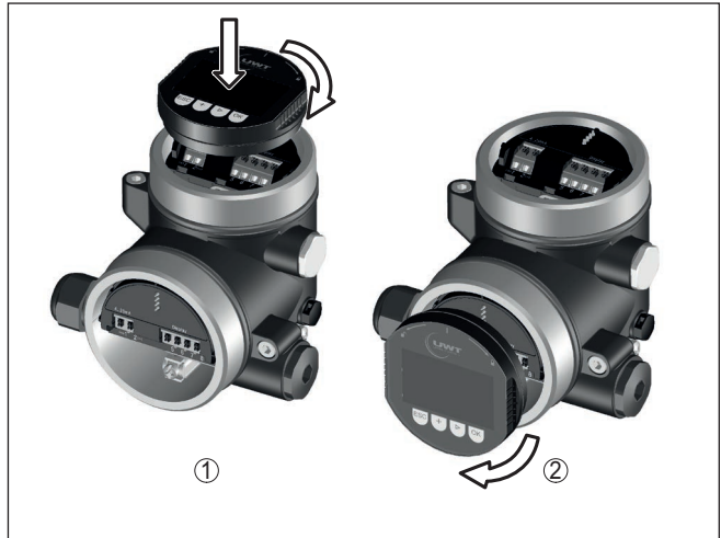
插图. 18: 将显示和调整模块装到双腔式壳体上
