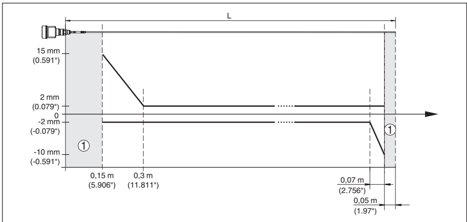
插图. 27: 棒型 NivoGuide 8100 在介质“油”中的测量偏差
