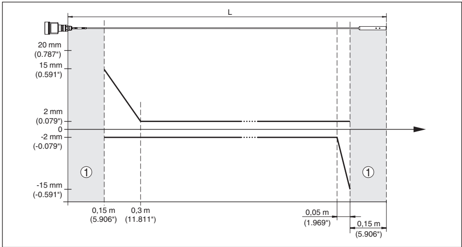
插图. 30: 绳型 (ø 4 mm/0.157 in) NivoGuide 8100 在介质“油”中的测量偏差
