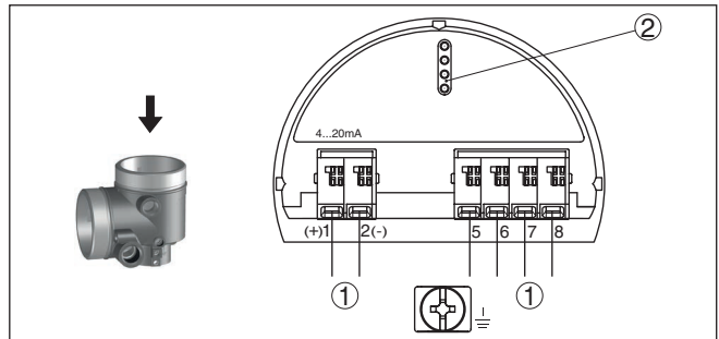
插图. 15: 双腔式壳体的电子部件腔
