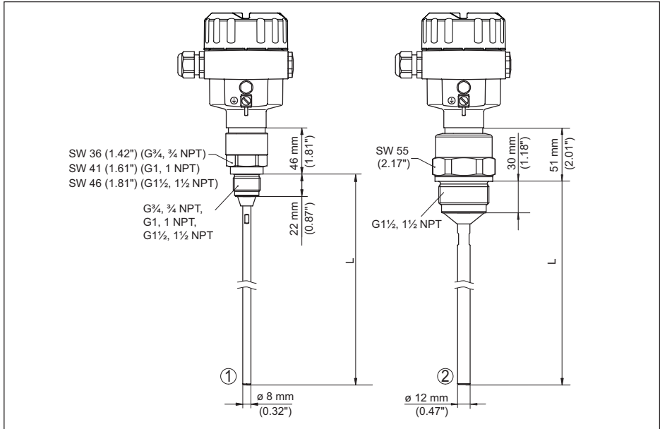
插图. 38: NivoGuide 8100, 螺纹型
