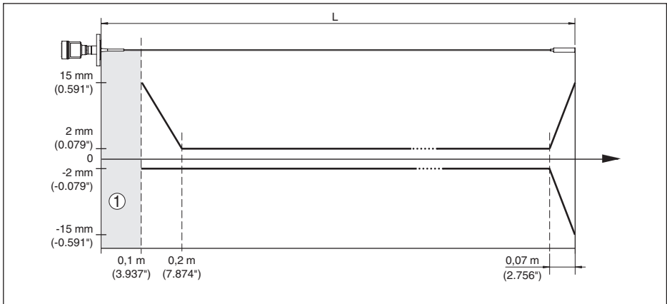
插图. 31: 在介质水中, 绳型 NivoGuide 8100 (ø 4 mm/0.157 in, 经 PFA 涂层) 的测量偏差
