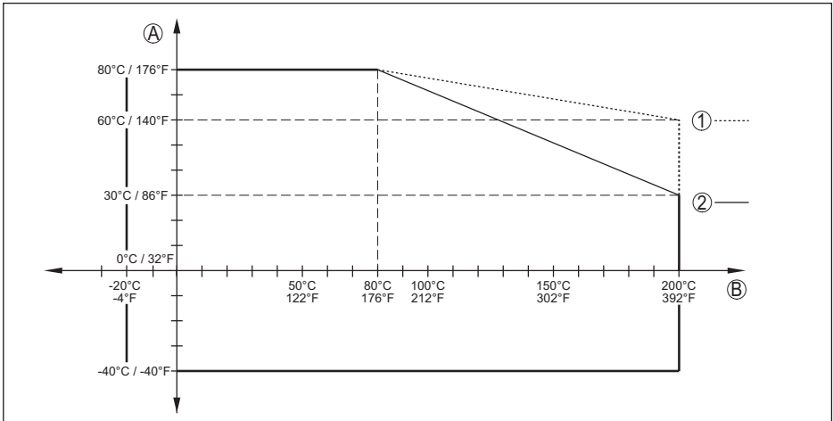
插图. 34: 环境温度 - 过程温度、带有温度连接元件的类型
