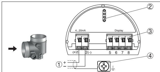
插图. 16: 双腔式壳体的接线腔
