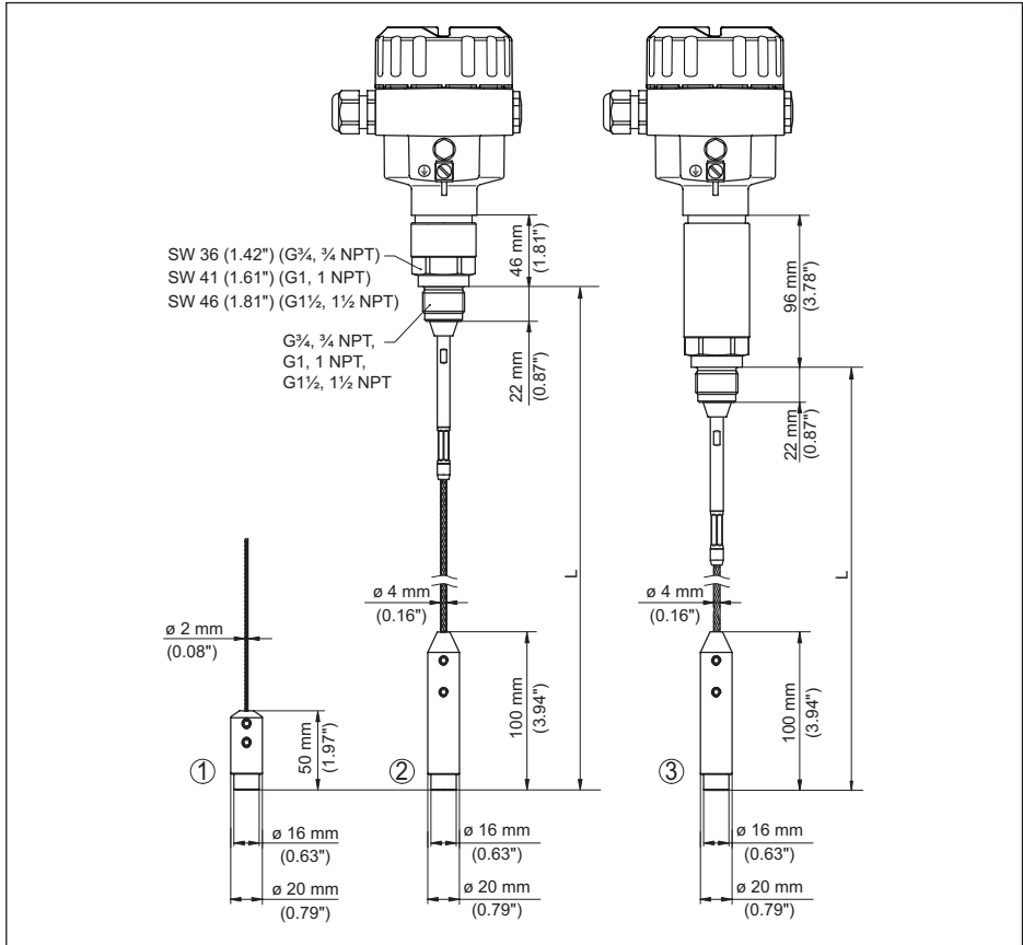
插图. 37: NivoGuide 8100, 带铅锤 (所有铅锤都带有用于环首螺钉的螺纹孔, M8) 的绳型
