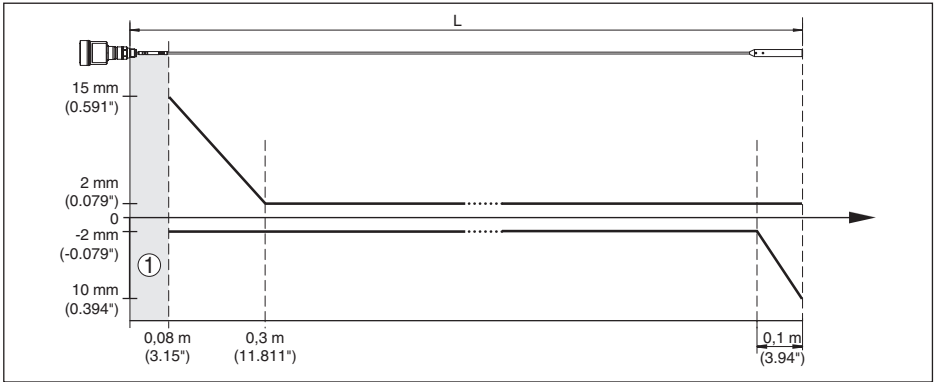
插图 28: 绳型 NivoGuide 8100 在介质“水”中的测量偏差
