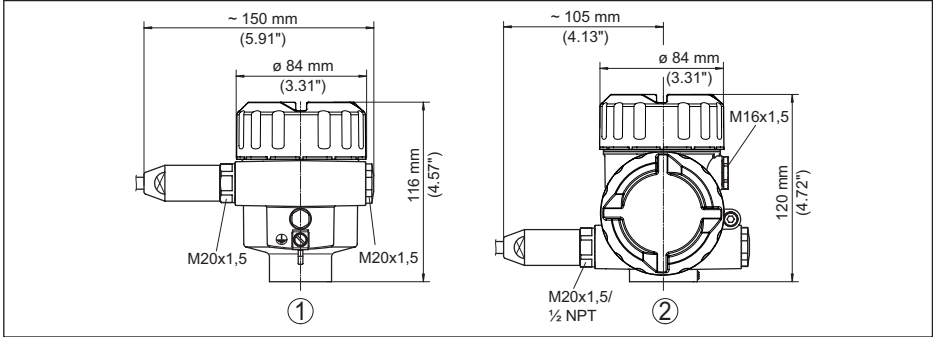
插图. 26: 采用保护等级达 IP 66/IP 68 (1 bar) 的壳体型式, (内装显示和调整模块后, 壳体高度增加了 9 mm/0.35 in)
