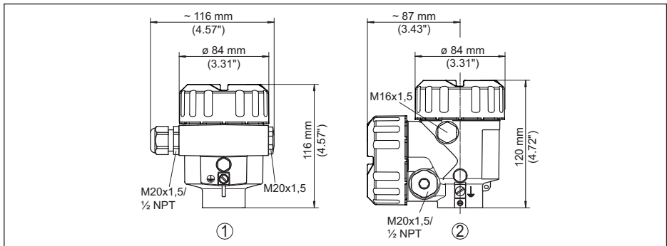
插图. 25: 采用保护等级达 IP 66/IP 68 (0.2 bar) 的壳体型式。(内装显示和调整模块后, 壳体高度增加了 9 mm/0.35 in)
