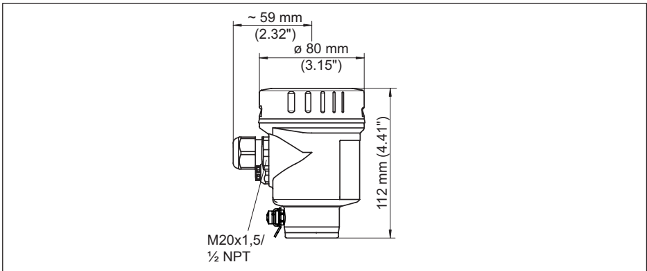
插图. 27: 采用保护等级达 IP 66/IP 68 (0.2 bar) 的壳体型式, (内装显示和调整模块后, 壳体高度增加了 9 mm/0.35 in)
