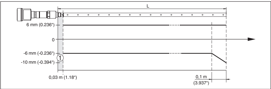
插图 21: 在介质“水”中同轴型 NivoGuide 8200 的测量偏差 (测量长度至 6 m/19.69 ft)
