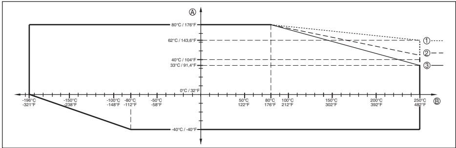
插图 24: 环境温度 - 过程温度, 标准型
