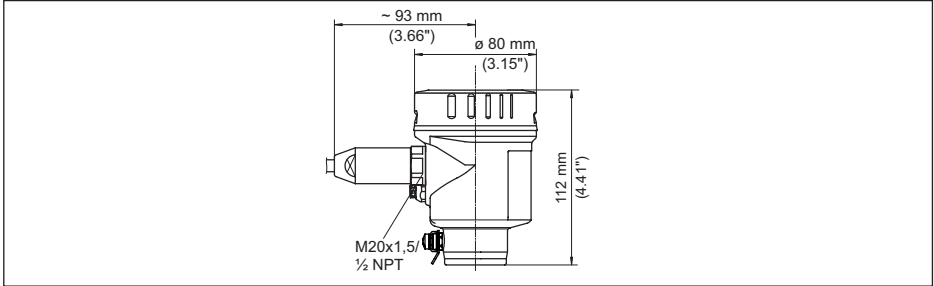
插图. 28: 采用保护等级达 IP 66/IP 68 (1 bar) 的壳体型式, (内装显示和调整模块后, 壳体高度增加了 9 mm/0.35 in)
