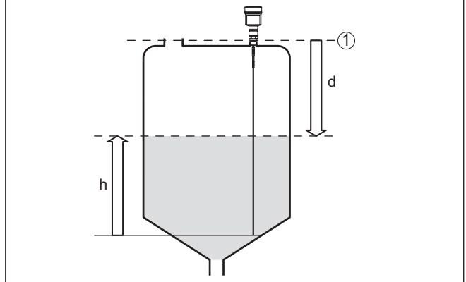
插图. 2: 物位测量
