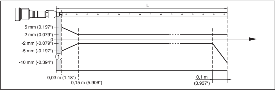
插图 20: 在介质“水”中同轴型的测量偏差 NivoGuide 8200 (测量长度至 1.5 m/4.92 ft)
