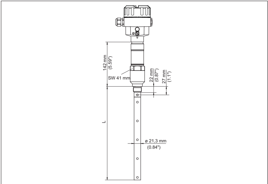
插图. 29: NivoGuide 8200, 带螺纹的同轴型 (-20 ... +250 °C/-4 ... +482 °F)
