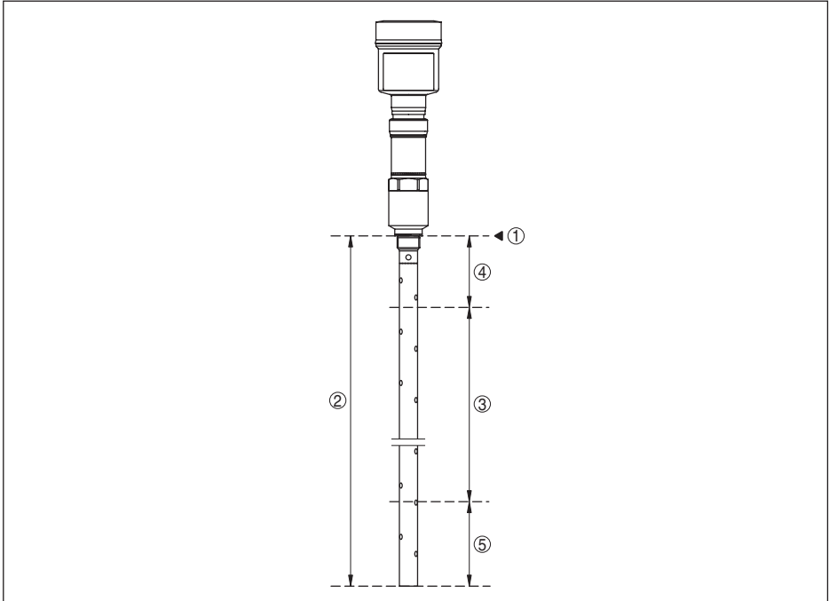
插图. 19: NivoGuide 8200 的测量范围
