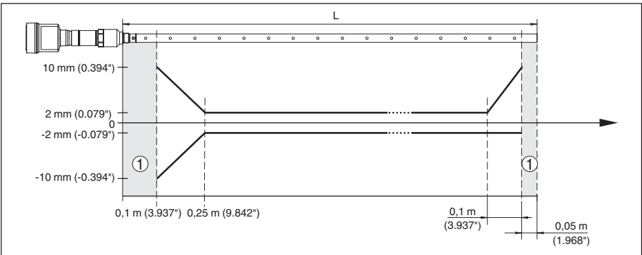
插图 22: 在介质“油”中同轴型 NivoGuide 8200 的测量偏差 (测量长度至 1.5 m/4.92 ft)
