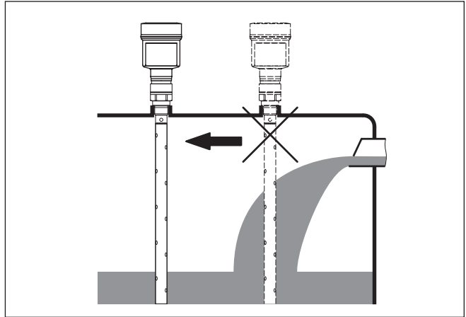
Fig. 5: Montagem do sensor no fluxo de entrada do produto
