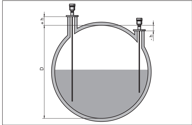
Fig. 14: Altura do reservatório e valor de correção da luva
