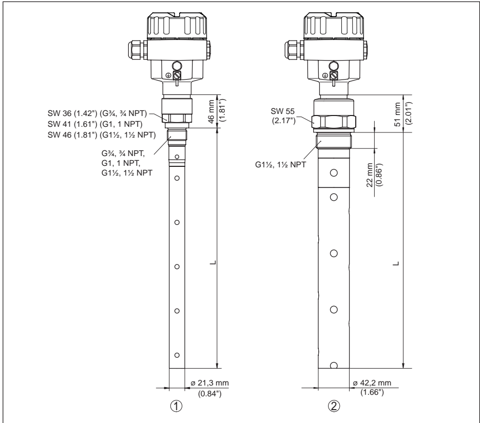
Fig. 32: NivoGuide 8100, Modelo com rosca
