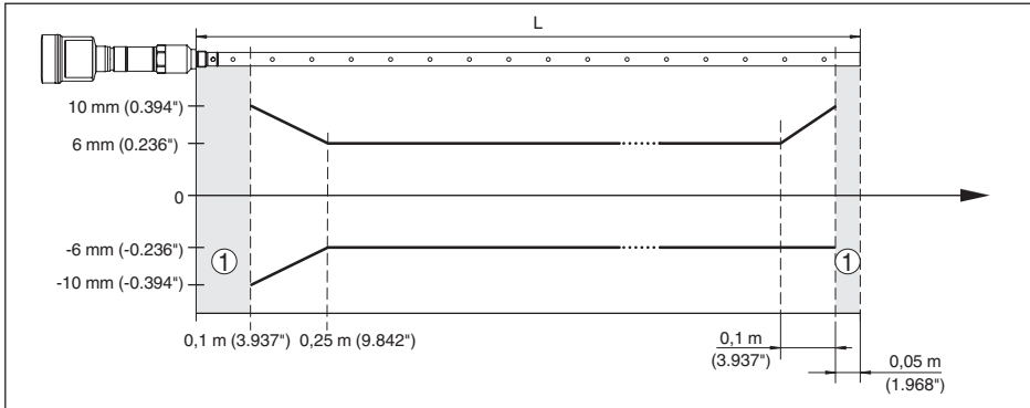
Fig. 22: Écart de mesure NivoGuide 8200 en version coaxiale dans l'huile (longueur de mesure jusqu'à 6 m/19.69 ft)
