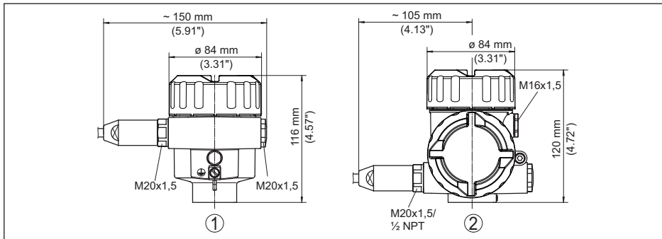
Fig. 25: Variantes de boîtier en protection IP 66/IP 68 (1 bar), (avec un module de réglage et d'affichage intégré, la hauteur du boîtier augmente de 9 mm/0.35 in)
