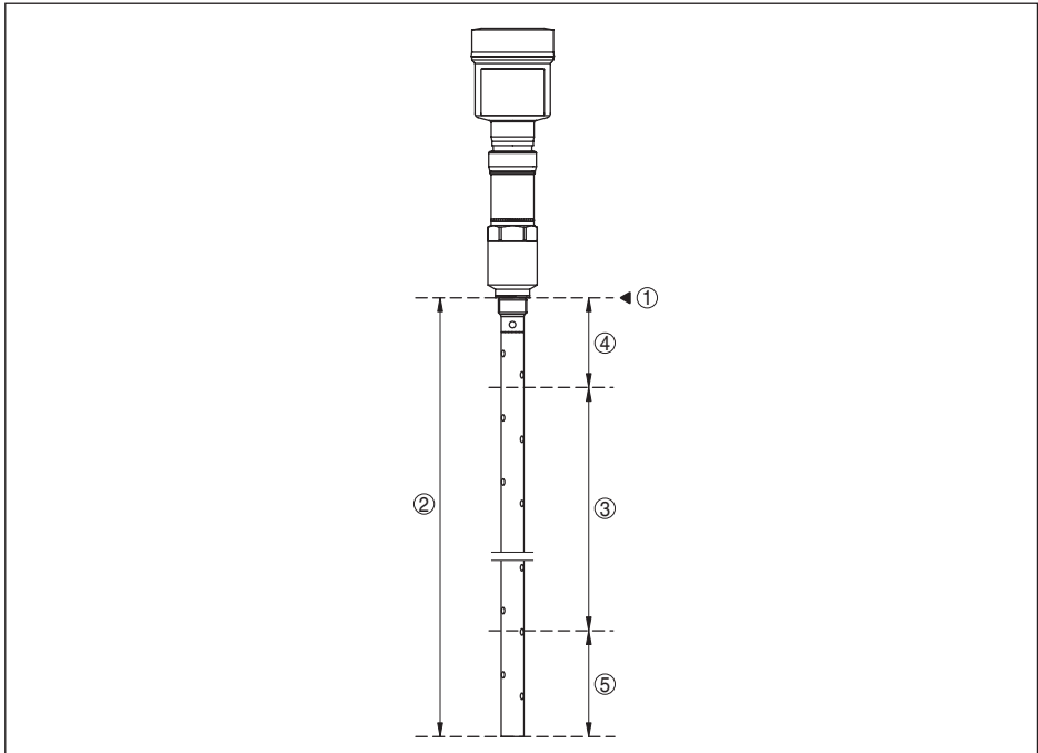
Fig. 18: Plages de mesure - NivoGuide 8200
