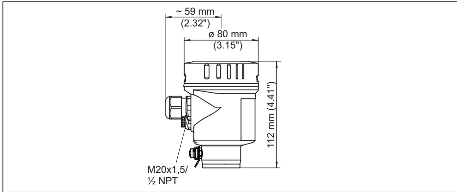
Fig. 26: Variantes de boîtier en protection IP 66/IP 68 (0,2 bar), (avec un module de réglage et d'affichage intégré, la hauteur du boîtier augmente de 9 mm/0.35 in)
