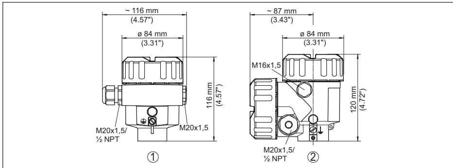
Fig. 24: Variantes de boîtier en protection IP 66/IP 68 (0,2 bar), (avec un module de réglage et d'affichage intégré, la hauteur du boîtier augmente de 9 mm/0.35 in)
