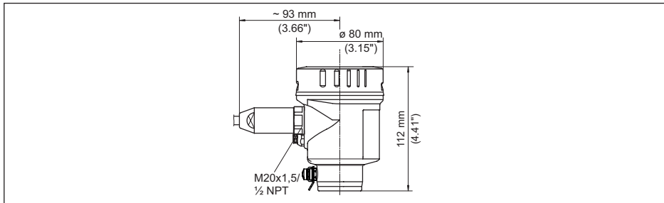
Fig. 27: Variantes de boîtier en protection IP 66/IP 68 (1 bar), (avec un module de réglage et d'affichage intégré, la hauteur du boîtier augmente de 9 mm/0.35 in)
