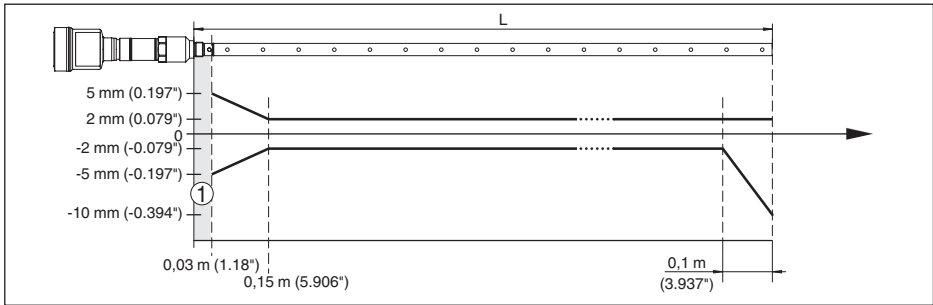
Fig. 19: Écart de mesure NivoGuide 8200 en version coaxiale dans l'eau (longueur de mesure jusqu'à 1,5 m/4.92 ft)
