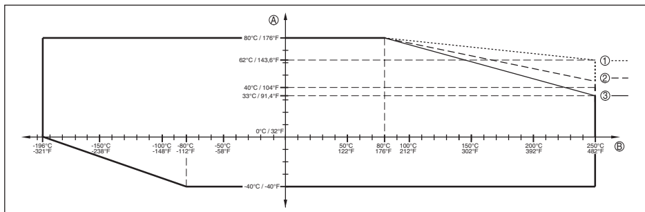
Fig. 23: Température ambiante - température process, version standard
