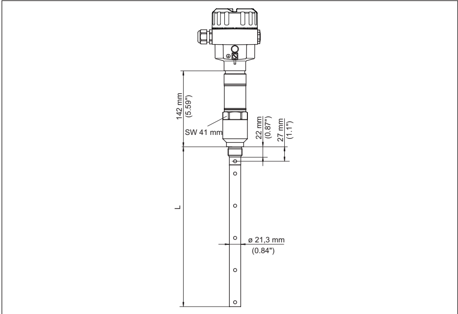
Fig. 28: NivoGuide 8200 - version coaxiale avec filetage (-20 ... +250 °C/-4 ... +482 °F)
