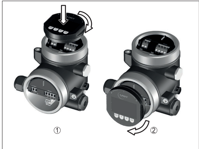
Fig. 13: Montage du module d'affichage et de réglage dans le boîtier à deux chambres
