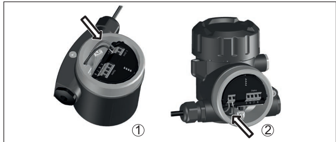
Abb. 3: Anschlusschritte 5 und 6
