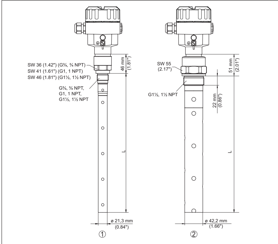
Abb. 24: NivoGuide 8100, Gewindeausführung
