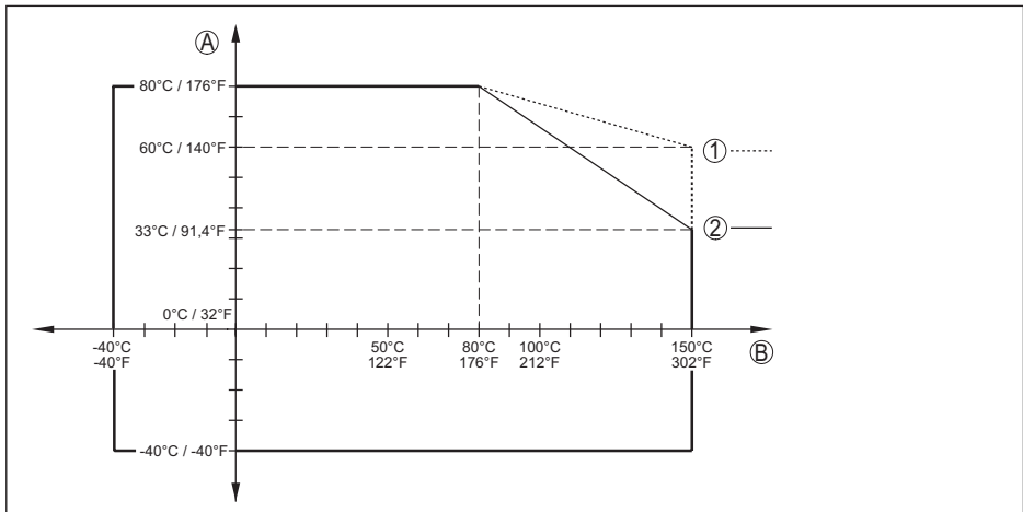
Abb. 20: Umgebungstemperatur - Prozesstemperatur, Standardausführung
