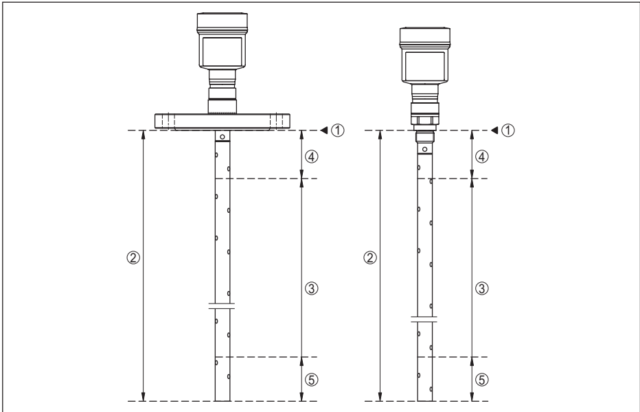
Abb. 17: Messbereiche - NivoGuide 8100
