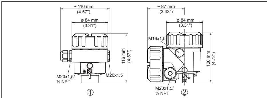
Abb. 22: Gehäuseausführungen in Schutzart IP 66/IP 68 (0,2 bar), (mit eingebautem Anzeige- und Bedienmodul vergrößert sich die Gehäusehöhe um 9 mm/0.35 in)
