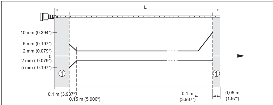
Abb. 19: Messabweichung NivoGuide 8100 in Koaxialausführung in Medium Öl
