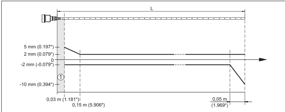
Abb. 18: Messabweichung NivoGuide 8100 in Koaxialausführung in Medium Wasser
