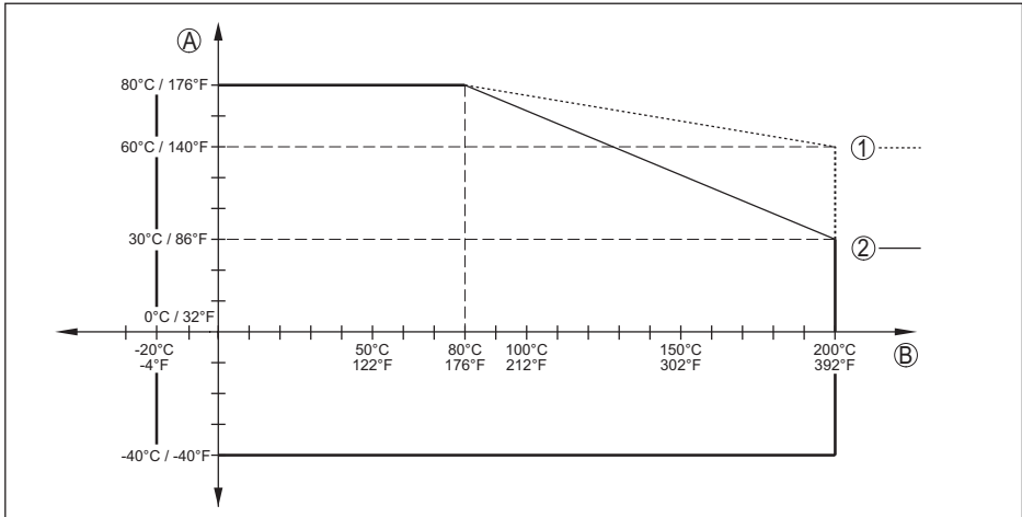
Abb. 21: Umgebungstemperatur - Prozesstemperatur, Ausführung mit Temperaturzwischenstück
